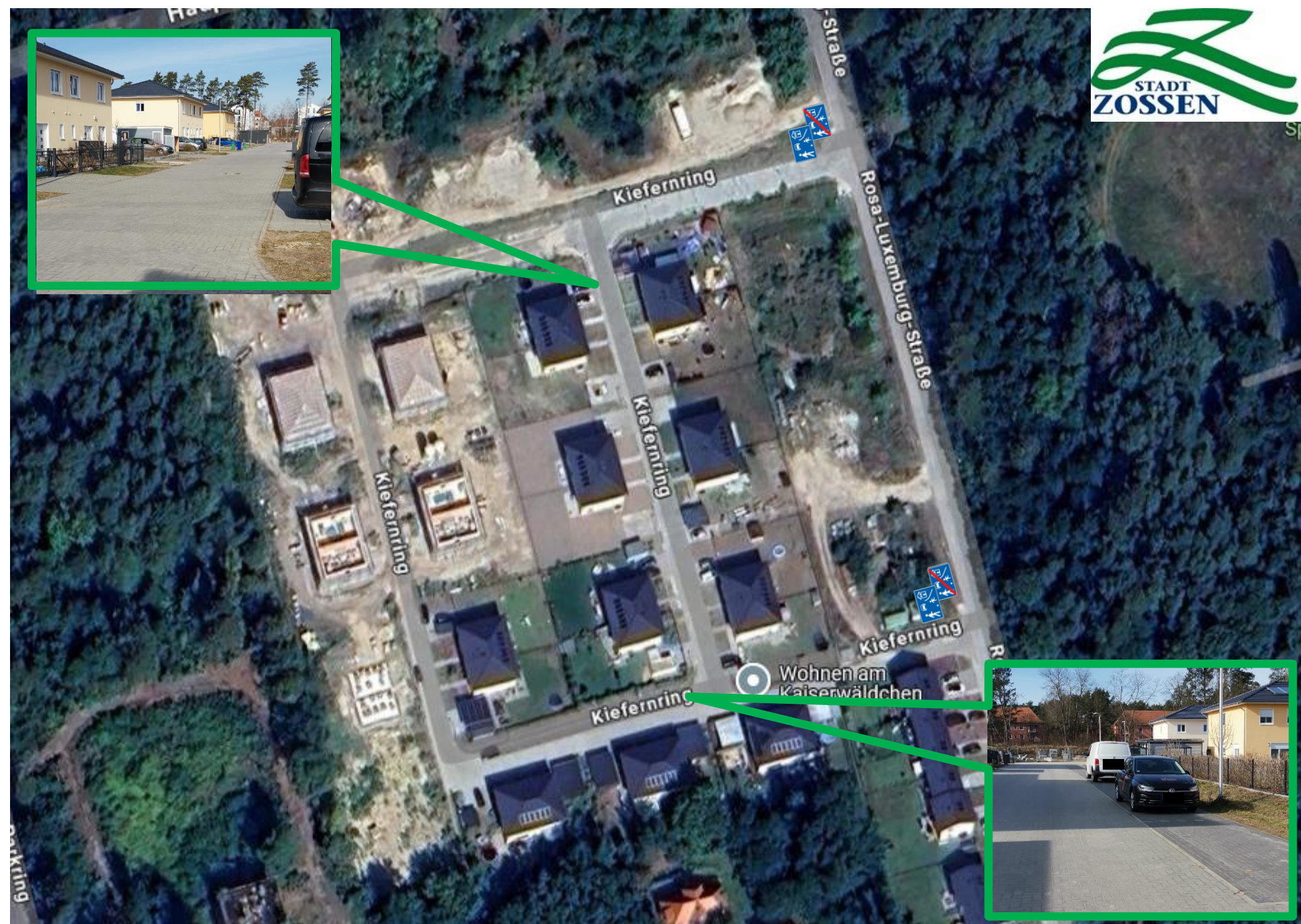
Einrichtung verkehrsberuhigter Bereich, Kiefernring in Waldstadt
